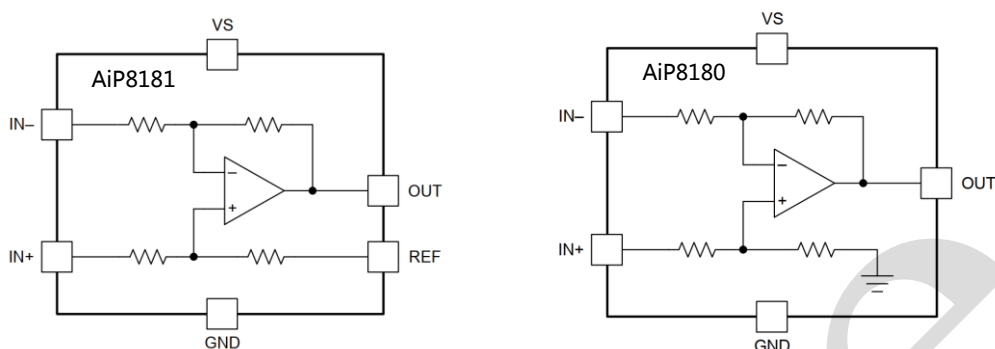
图 1 AiP8181 与 AiP8180 功能框图
