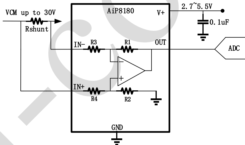
图10 AiP8180典型应用线路
