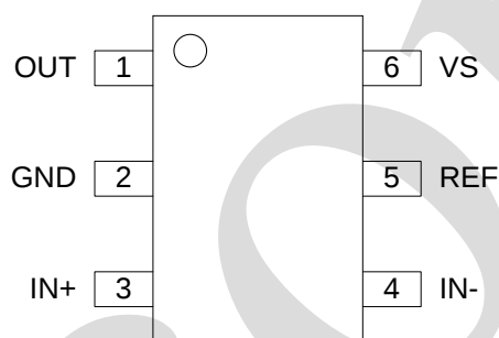
图 2 AiP8181 引脚排列图
