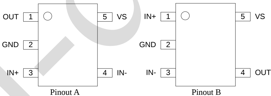
图 3 AiP8180 引脚排列图
