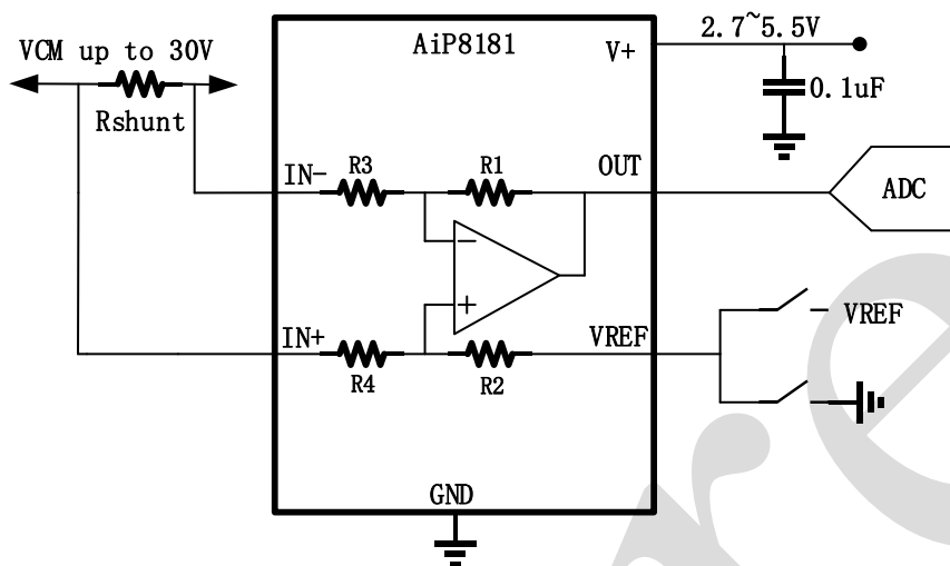
图9 AiP8181典型应用线路
