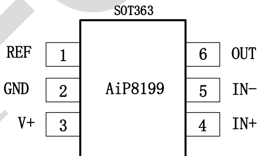
AiP8199 引脚排列图
