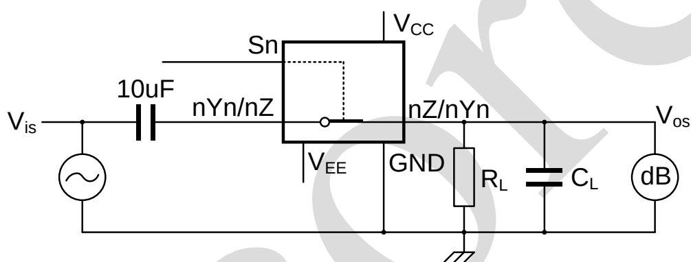
a. Test circuit
